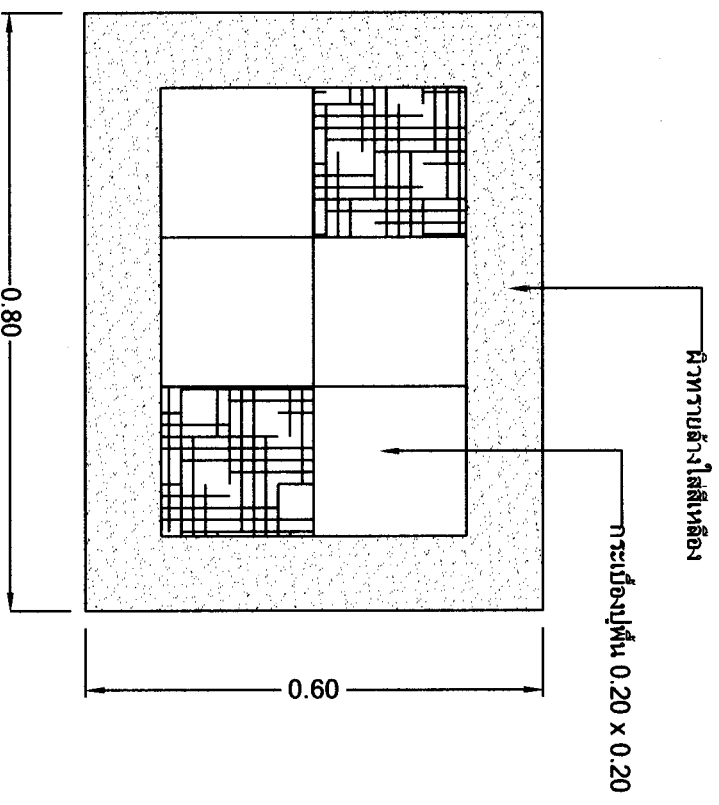
แปลนพื้น 1:10
